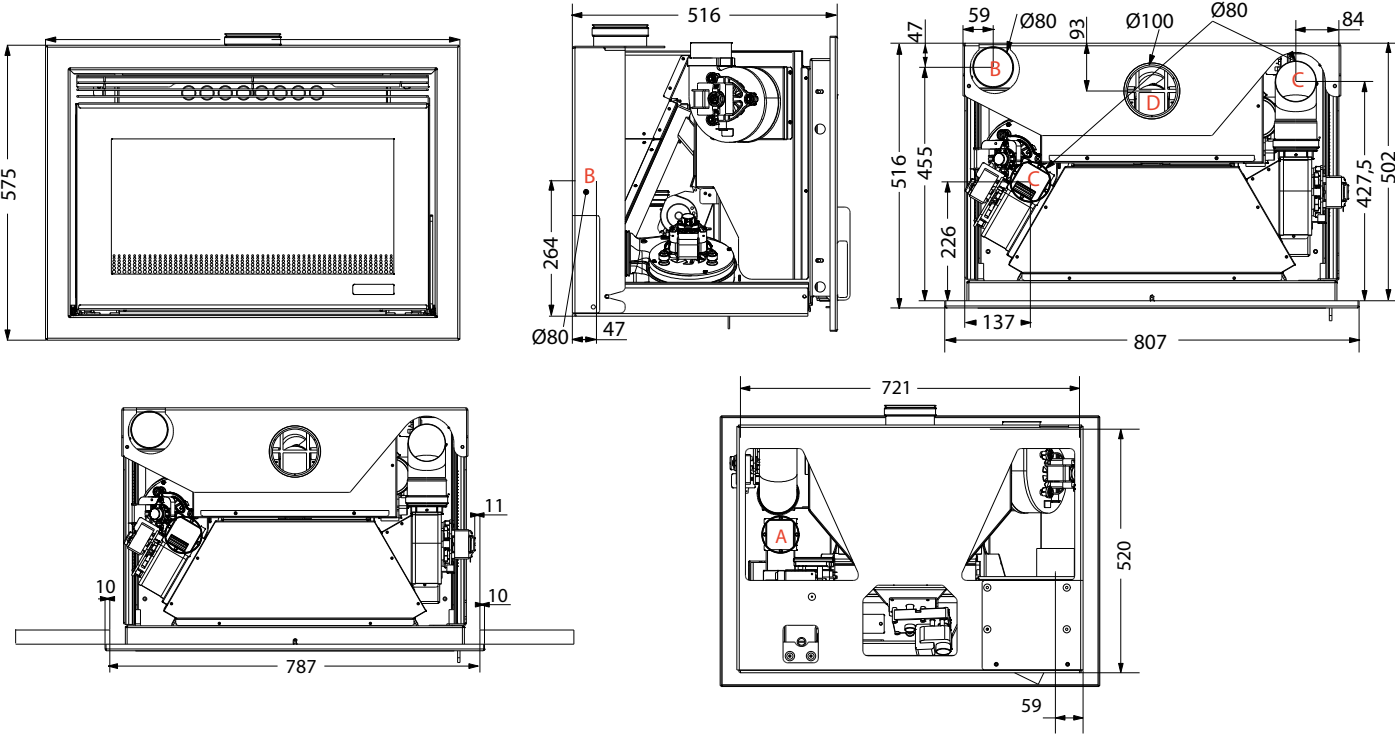
Mini Ory AP 700 con cassetto di carico pellet frontale compreso di cornice estetica / Mini Ory AP 700with pellet loading tray with aesthetic frame / Mini Ory AP 700 avec le tiroir de remplissage pellet compris le cadre esthétique/ Mini Ory AP 700 con el cajón de llenado de pellet frontal completo de marco estetico
